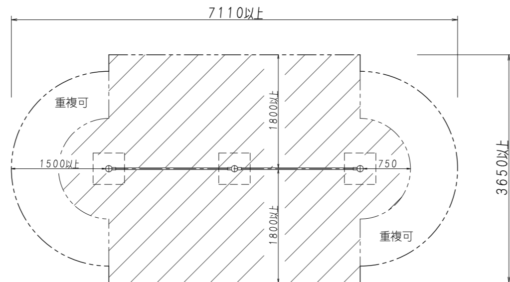
平面図 S = 1/60
