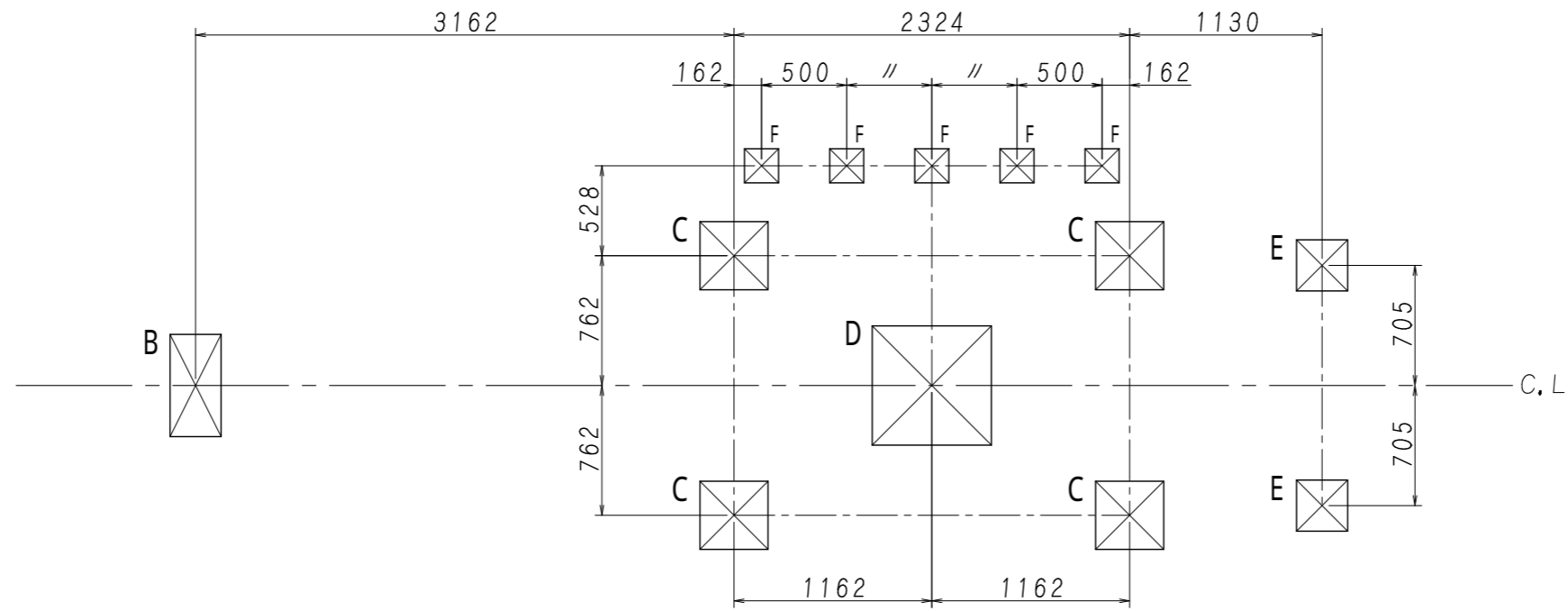
基礎平面図 S = 1/40
