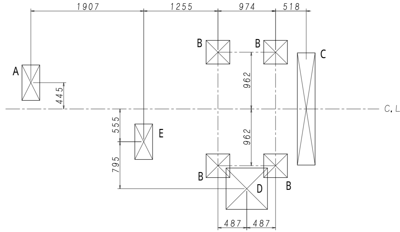
基礎平面図 S = 1/40
